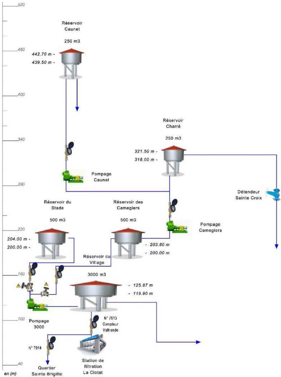
Profil hydraulique du réseau d'alimentation en Eau Potable sur Ceyreste
