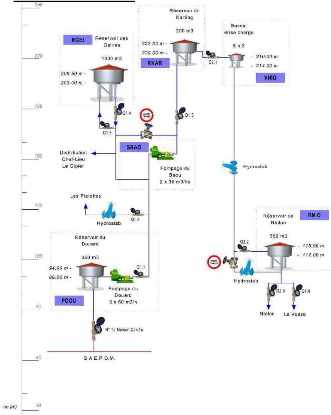
Profil hydraulique du réseau d’alimentation en eau potable du Rove
