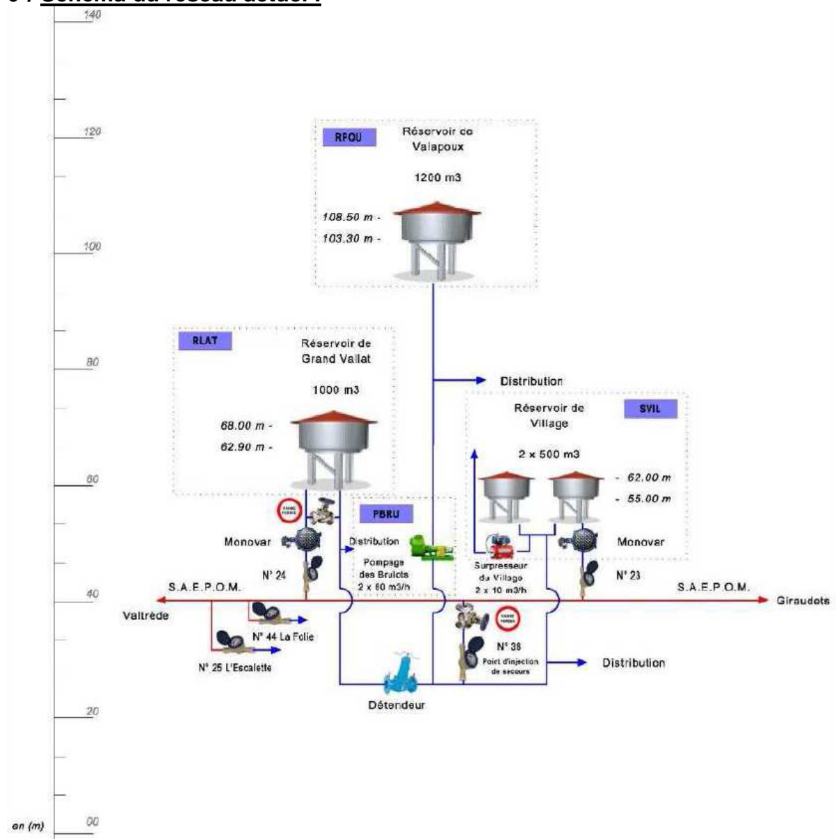
Profil hydraulique du réseau d'alimentation en eau potable sur Sausset-les-Pins
